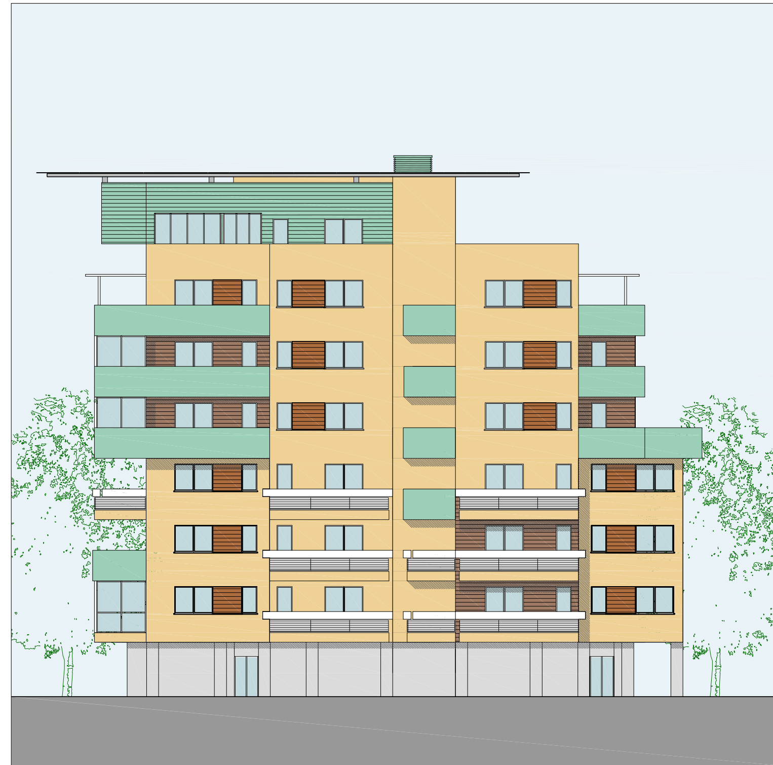
Prospetto tipo
